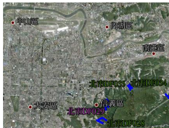
圖 2-2-2、土石流潛勢溪流位置圖
